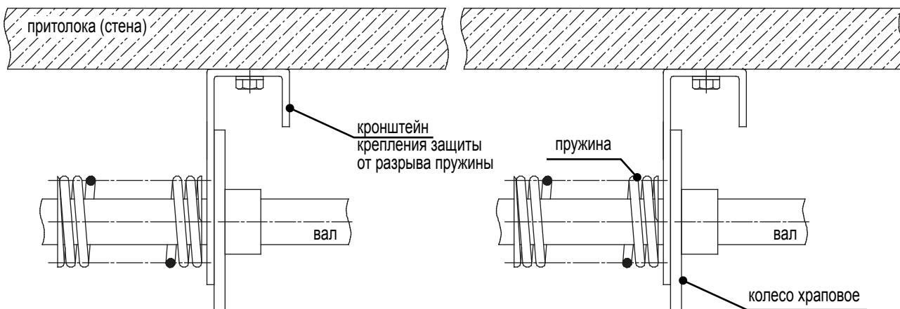
ВАРИАНТ КРЕПЛЕНИЯ ДВУХ ЛЕВЫХ ПРУЖИН С ЗАЩИТАМИ ОТ РАЗРЫВА ПРУЖИН
