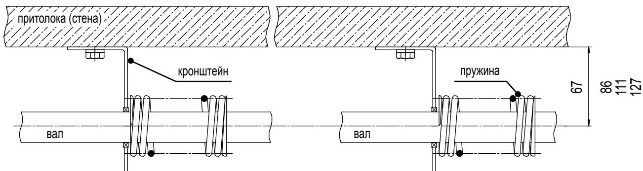
ВАРИАНТ КРЕПЛЕНИЯ ДВУХ ПРАВЫХ ПРУЖИН С ЗАЩИТАМИ ОТ РАЗРЫВА ПРУЖИН
