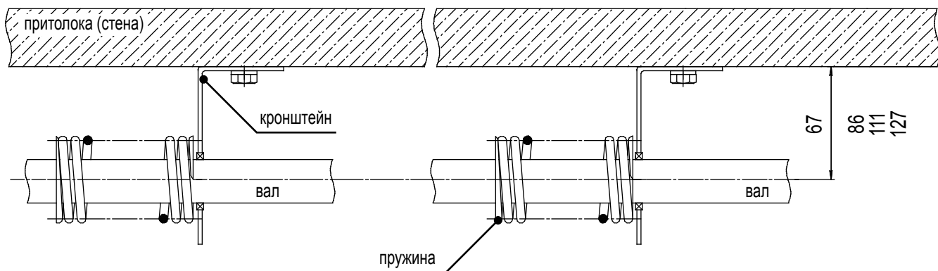
ВАРИАНТ КРЕПЛЕНИЯ ДВУХ ЛЕВЫХ ПРУЖИН
